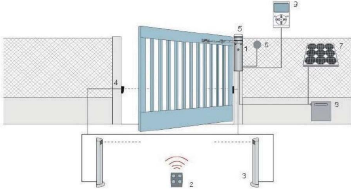
1) Walky 2) Uzaktan Kumanda Vericisi 3) Ayaklı Emniyet Fotoseli 4) Emniyet Fotoseli 5) Flaşör 6) Dijital ya da Anahtarlı Şartel 7) Syp Güneş Enerji Sistemi 8) Acil Durum Bataryası 9) O-view
